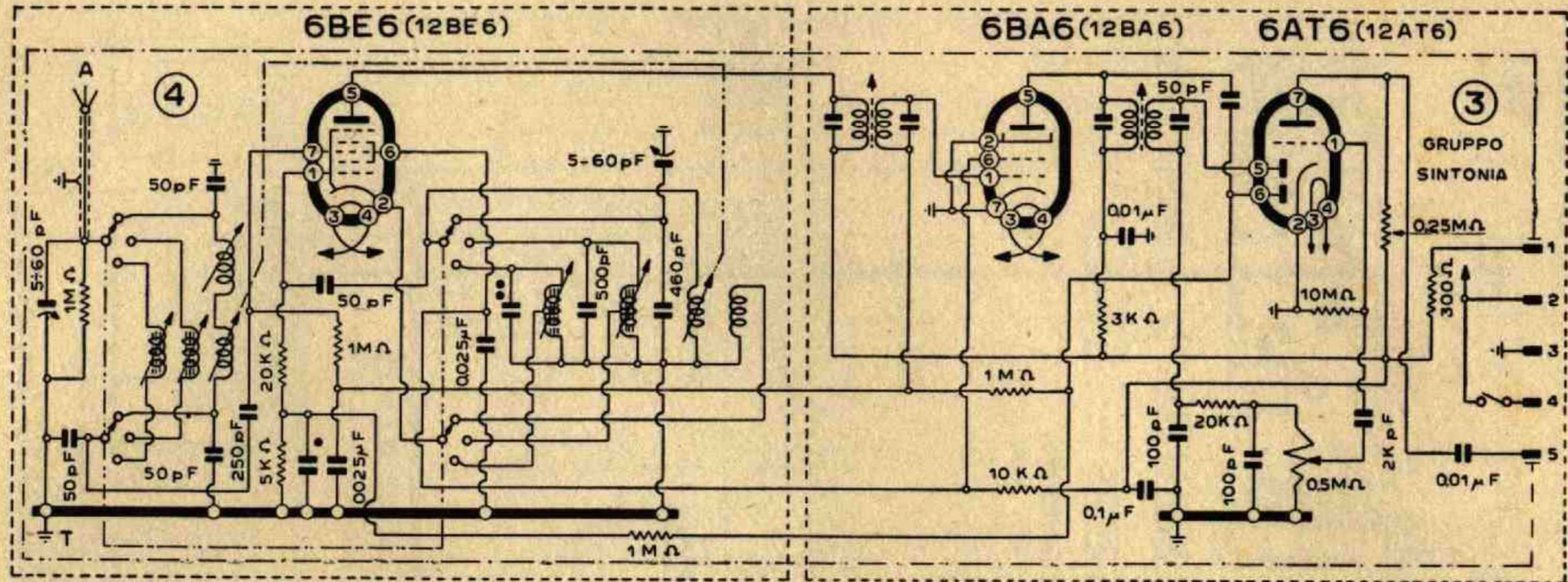
GRUPPO DEI FILAMENTI GRUPPO SINTONIA 6BE6 6BA6
